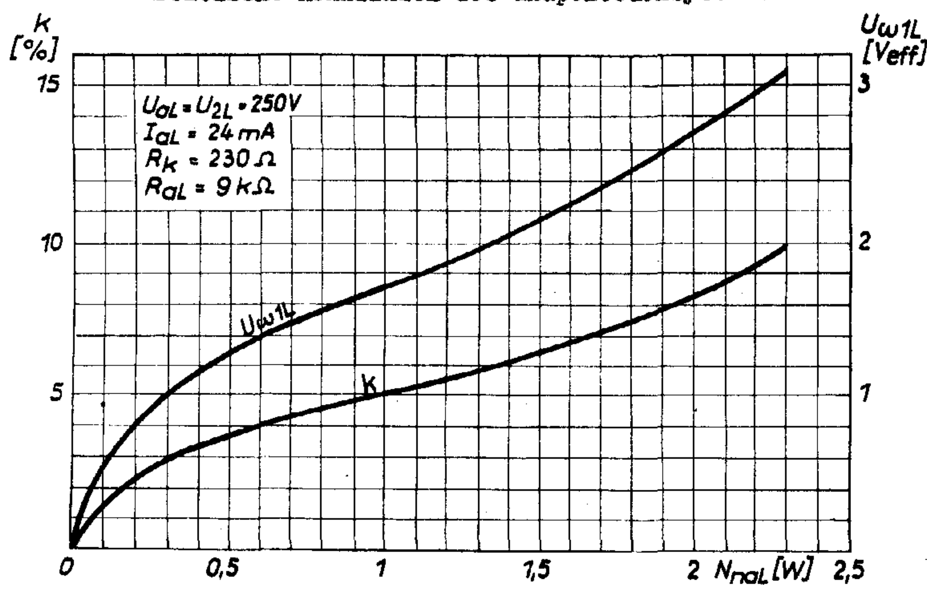
Eingangswechselspannung und Klirrfaktor als Funktion der Ausgangsnutzleistung
