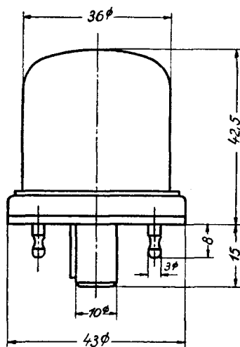
Kolbenabmessungen
