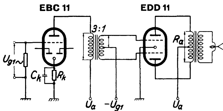
Prinzipschaltbild
