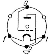
Sockelschaltenschema
