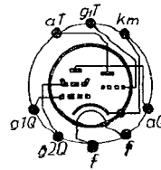
Sockelschaltungschema
