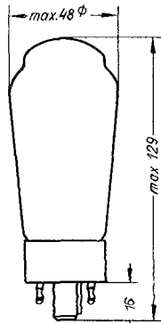
Kolbenabmessungen
