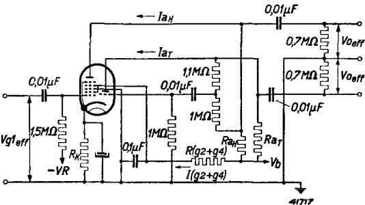
Fig. 4 Schakeling van ECH 4 als faseomkeerbuis met tegenkoppeling, ter verklaring van de bovenstaande omschrijvingen en symbolen.
