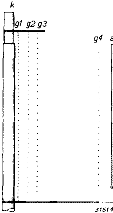
Abb. 4 Senkrechter Schnitt durch das Elektroden-system des Hexodenteiles (Schnitt A-B der Abb. 3).
