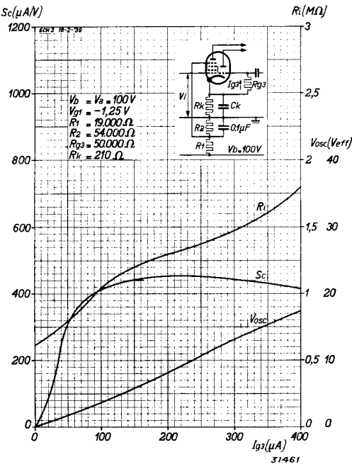
Abb. 14 Mischsteilheit S_c , Innenwiderstand R_i und effektive Oszillatorwechselspannung V_{osc} als Funktion des Oszillatorgitterstroms I_{g3} bei R_{g3} = 50.000 \text{ Ohm} , V_a = 100 \text{ V} und Schirmgitterspeisung über einen Spannungsteiler von 19.000 + 54.000 \text{ Ohm} (für umschaltbare G/W-Geräte).
