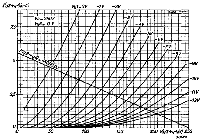
Fig. 17 Schermroosterstroom als functie van de schermroosterspanning, bij V_a = 250V en V_{g_1} = 0V , met de negatieve roosterspanning als parameter.
