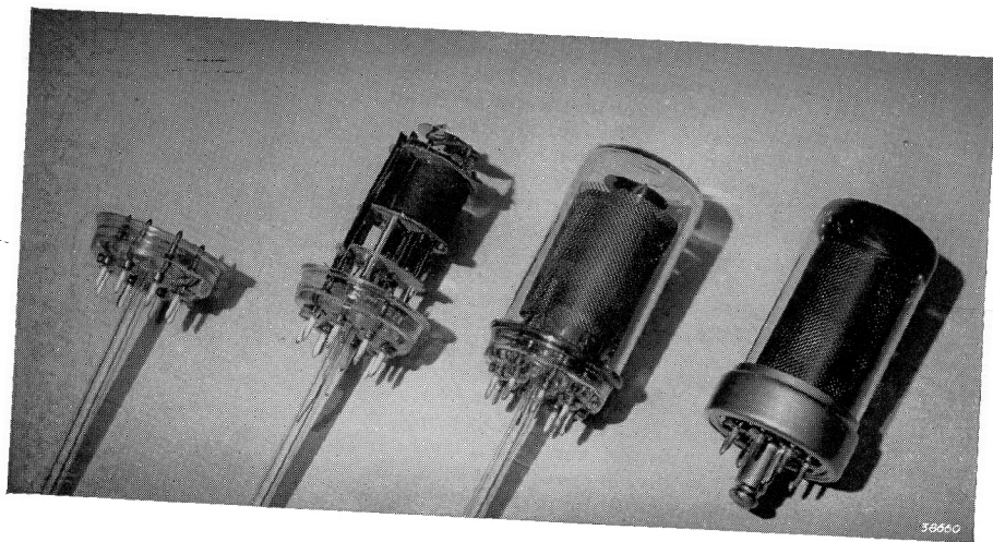
Fig. 1 Vier stadia uit de montage van de triode-heptode sleutelbuis ECH 21
