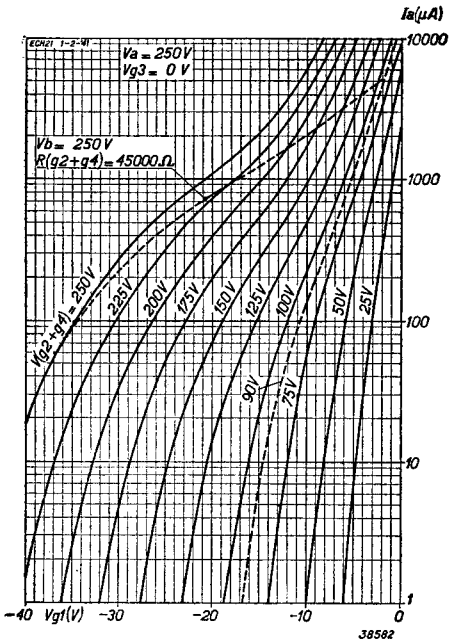
Fig. 12 Toepassing van het heptodegedeelte als m.f. versterker. Anodestroom als functie van de negatieve roosterspanning bij V_a = 250 \text{ V} en V_{g3} = 0 \text{ V} , met de schermroosterspanning als parameter.
