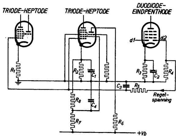
Fig. 5 Vereenvoudigd schema voor het verkrijgen van de negatieve rooster-spanning en de spanning voor de automatische volumeregeling, bij gebruik van de buizen ECH 21 en EBL 21; de vertragingsspanning van de automatische volumeregeling wordt hierbij op de juiste waarde ingesteld. Hiertoe wordt de spanningval over den kathodeweerstand R_k van de eindbuis gebruikt. De stroom, die door den potentiometer voor de schermroostervoeding vloeit, loopt ook door den kathodeweerstand van de tweede ECH 21, zoodat de spanningval over dezen weerstand ( R_k ) nagenoeg onafhankelijk is van de regeling van het heptedegedeelte.
