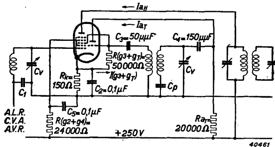
Fig. 7 Principele schakeling voor toepassing van de ECH 21 als mengbuis
