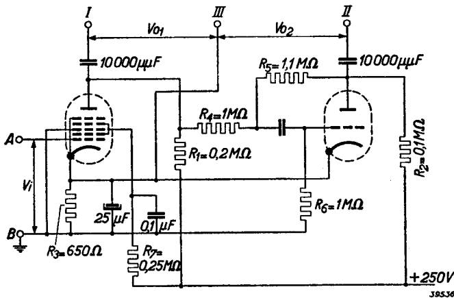
Fig. 6 Principiele schakeling van de ECH 21 als L.F. versterkerbuis en faseomkeerbuis vóór een balanseindtrap. De uitgangspanningen V_0 en V_{0a} zijn bij deze schakeling zuiver in tegenfase en worden aan de roosters van twee in balans geschakelde eindbuizen geleid. Terwille van de duidelijkheid zijn het triode- en het heptodegedeelte afzonderlijk getekend.
