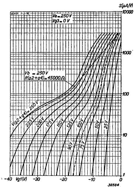
Fig. 13 Steilheid als functie van de negatieve roosterspanning van het heptodegedeelte bij V_a = 250 \text{ V} en V_{g3} = 0 \text{ V} , met de schermroosterspanning als parameter.
