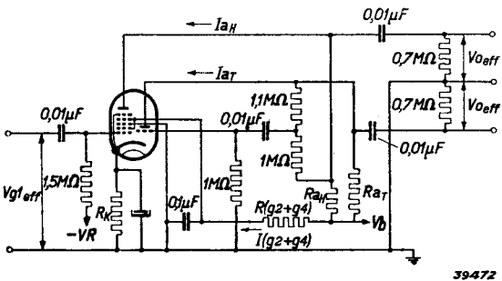
Fig. 16 Schakeling van de ECH 21 als faseomkeerbuis met tegenkoppeling, ter verklaring van de bovenstaande omschrijvingen en symbolen.
