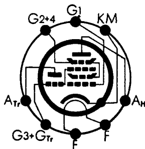
Sockelschaltbild
