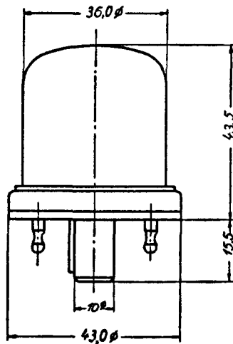
Kolbenabmessungen
