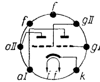
Sockelschaltungsdiagramm
