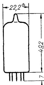
max. Abmessungen
