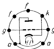
Sockelschalt-schema
