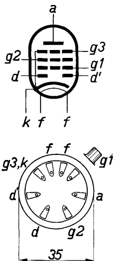
Schematische voorstelling van de duo-diode-penthode EBL 1, benevens schema van aansluiting der electroden aan de huls. Het stuurrooster is met de top-aansluiting van den ballon verbonden.
