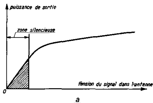
a) Courbe représentative de la puissance modulée en fonction de la tension du signal d'un réglage automatique différé (courbe de C.A.V.). La partie hachurée représente la zone silencieuse du réglage silencieux. Le mutisme y est supprimé avant le commencement du réglage automatique.
