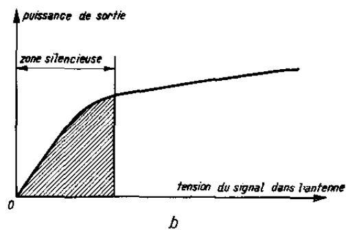
b) La même courbe que celle de a). Le mutisme y est supprimé après le commencement du réglage automatique.
