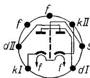
Sockelschaltchema
