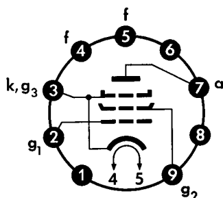
Sockelschaltbild Base connection
