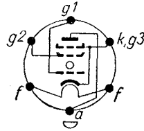
Sockelschaltschema
