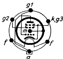
Sockelschaltschema
