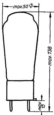
Kolbenabmessungen
