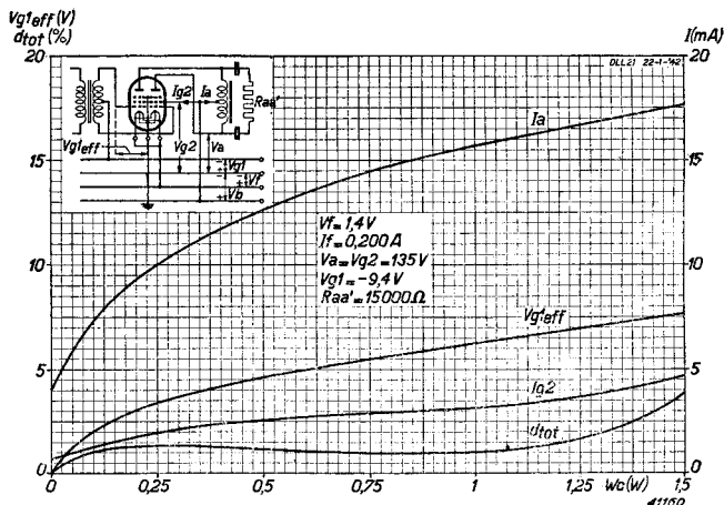
Fig. 13 Totale anodestroom en schermroosterstroom, totale vervorming en verciachte roosterwisselspanning per rooster als functie van het geleverde vermogen bij V_b = V_a = V_{g_2} = 135 V, V_f = 1,4 V, I_f = 200 mA, bij klasse B balansschakeling
