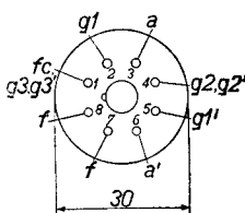
Fig. 2 Rangschikking van de elektroden en aansluitingen van de huls.
