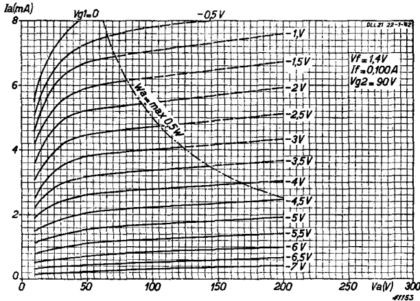
Fig. 5 Anodestroom van een penthodegedeelte als functie van de anodespanning bij V_{g1} = 90V , V_f = 1,4V en I_f = 100mA , met V_{g2} als parameter.
