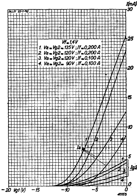
Fig. 4 Anode- en schermroosterstroom van een penthodegedeelte der DLL 21 als functie van de negatieve roosterspanning, bij V_f = 1,4V , voor verschillende waarden van de anode- en schermroosterspanning en van de gloeistroom.
