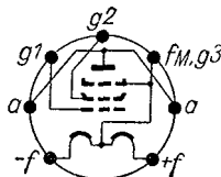
Sockelschaltchema
