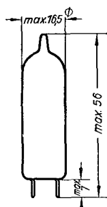
Kolbenabmessungen
