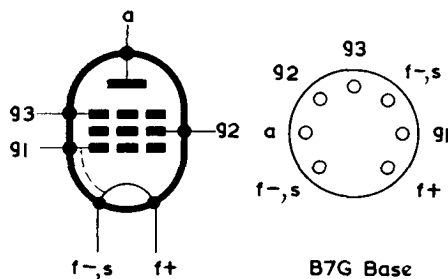
B7G Base
