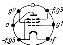
Sockelschaltchema
