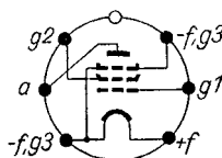
Sockelschaltschema
