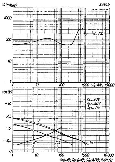
Fig. 8 Bovenste kromme: Effectieve waarde van de roosterwisselspanning als functie van de steilheid voor 1% kruismodulatie, bij V_a = V_b = 90 V. Onderste krommen: Steilheid S , anodestroom I_a , schermroosterstroom I_{g_2} en inwendige weerstand R_i als functie van de neg. roosterspanning V_{g_1} , bij V_a = V_{g_2} = 90 V.
