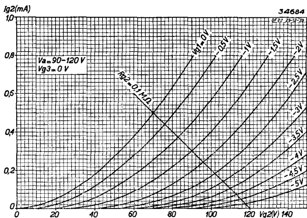
Fig. 6 Schermroosterstroom als functie van de schermroosterspanning, bij V_a = 90-120 V, met V_{g_1} als parameter.
