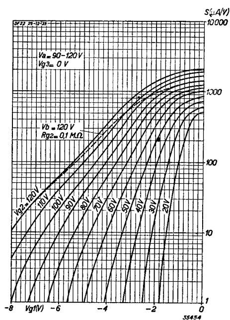
Fig. 4 Steilheid als functie van de negatieve rooster- spanning, bij V_a = 90-120 V , met V_{g3} als para- meter. De gestippelde kromme geldt voor een geregelde buis bij voeding van het schermrooster via 0,1 M\Omega uit de 120 V spanningbron.
