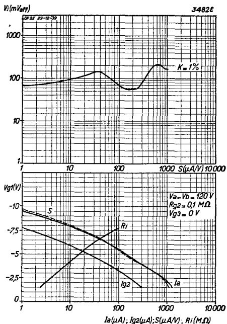
Fig. 7 Bovenste kromme: Effectieve waarde van de roosterwisselspanning als functie van de steilheid voor 1% kruismodulatie, bij V_a = V_b = 120 V. Onderste krommen: Steilheid S , anodestroom I_a , schermroosterstroom I_{g_2} en inwendige weerstand R_i als functie van de neg. roosterspanning V_{g_1} , bij V_a = V_b = 120 V.
