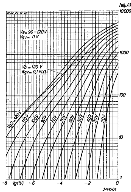
Fig. 3 Anodestroom als functie van de negatieve rooster- spanning, bij V_a = 90-120 V , met V_{g3} als para- meter. De gestippelde kromme geldt voor een geregelde buis bij voeding van het schermrooster via 0,1 M\Omega uit de 120 V spanningbron.
