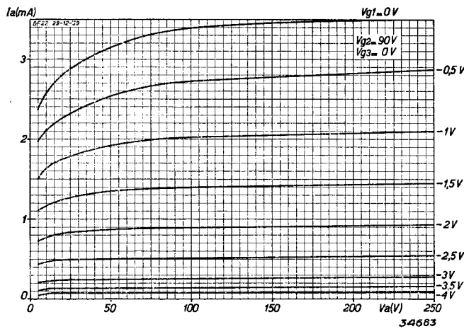
Fig. 5 Anodestroom als functie van de anodespanning, bij V_{g2} = 90 V , met V_{g1} als parameter.
