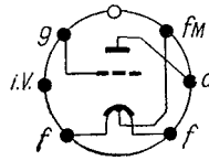
Sockelschaltschema
