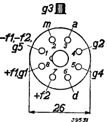
Fig. 2 Rangschikking van de elektroden en aansluitingen van de huls.
