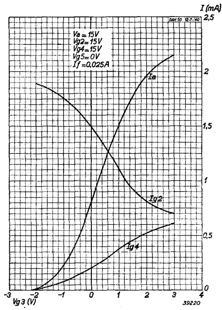
Fig. 4 Anodestroom, stroom van het ruimteladingrooster en schermroosterstroom als functie van de negatieve spanning aan rooster 3 (stuurrooster), bij V_{g2} = V_{g4} = 15 \text{ V} .
