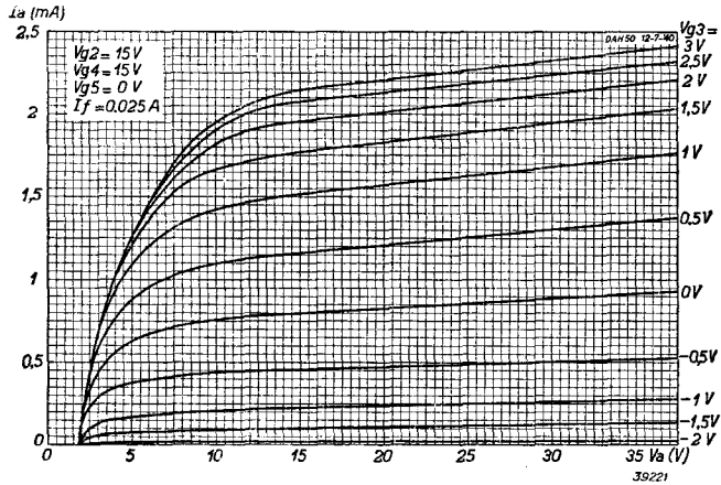
Fig. 5 Anodestroom als functie van de anodespanning, met V_{g3} als parameter.
