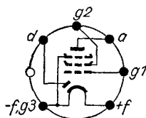
Sockelschaltchema
