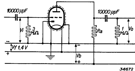
Fig. 3 Schakeling ter verklaring van de bij de dynamische gegevens vermelde symbolen.
