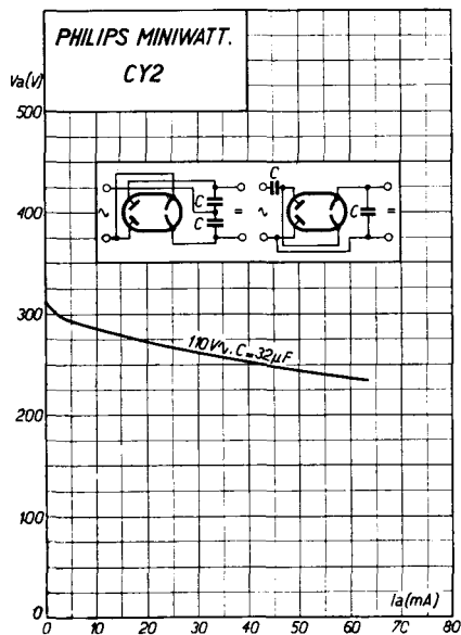
Belastungskennlinie der Röhre CY 2 als Spannungsverdoppler.
