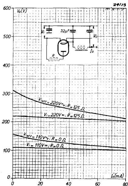
Abb. 3 Belastungskennlinien der Röhre CY 1.
