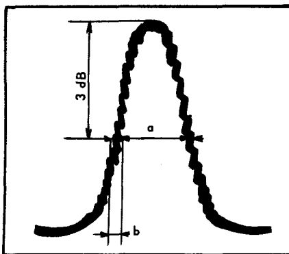
F_m \simeq 5 kHz, \Delta F = 1.400 \times \frac{b}{a} \simeq 150 kHz défaut caractérisé
