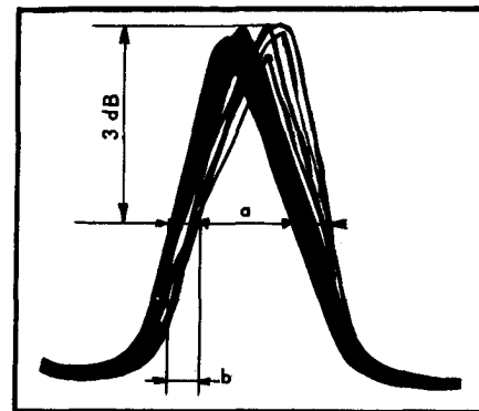
F_m = 35 Hz, \Delta F = 1.400 \frac{b}{a} = 300 kHz défaut caractérisé
