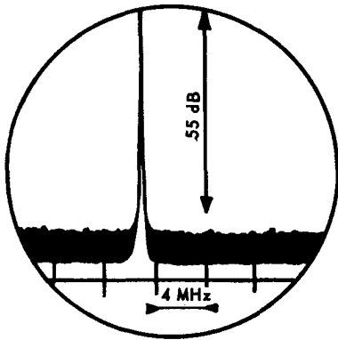
Exemple d'oscillogramme observé à l'analyseur de spectre
