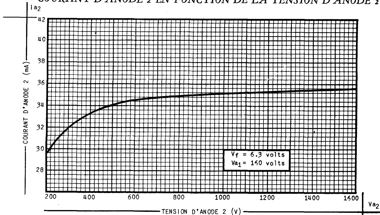
COURANT D'ANODE 2 EN FONCTION DE LA TENSION D'ANODE 2
