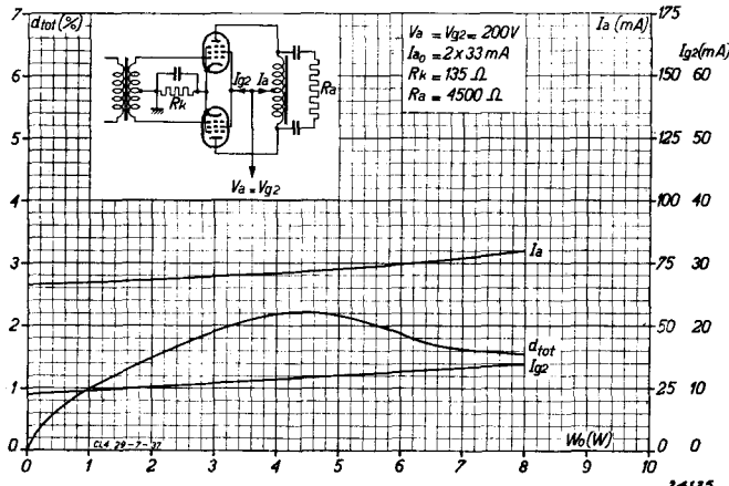
Abb. 6 Anodenstrom, Schirmgitterstrom und Gesamtverzerrung als Funktion der Ausgangsleistung bei Verwendung von zwei Röhren CL 4 als Gegentaktendverstärker.
