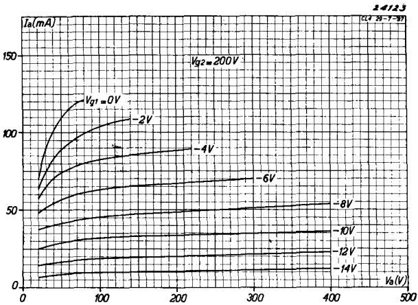
Abb. 4 Anodenstrom als Funktion der Anodenspannung bei V_{g3} = 20\text{ V} und verschiedenen negativen Gitterspannungen.
