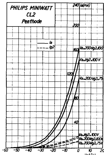
Anodenstrom und Schirmgitterstrom als Funktion der neg. Gitters.
