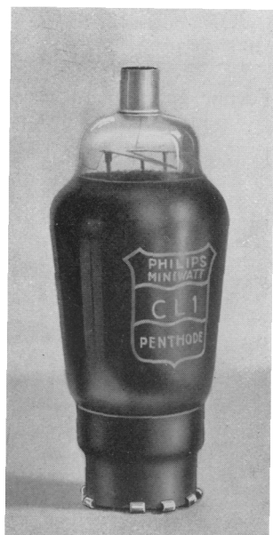
Die 5-Watt-Endpenthode der G/W-Serie.
