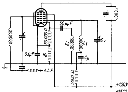
2834 Abb. 9 Speisung der Oszillatoranode über die Schwingspule mit Hilfe eines Serienwiderstandes von 5000 Ohm.
