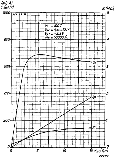
Innenwiderstand, Mischsteilheit und Oszillatorgitterstrom als Funktion der Oszillatorspannung bei einem Ableitwiderstand von 50.000 Ohm und bei V_a = 100 \text{ V} .
