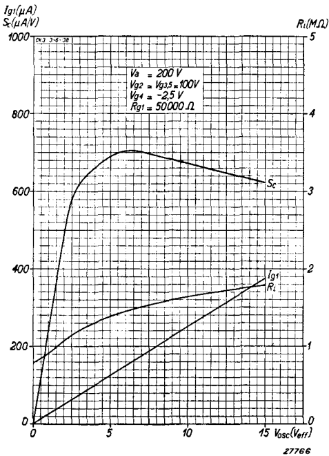
Innenwiderstand, Mischsteilheit und Oszillatorgitterstrom als Funktion der Oszillatorspannung bei einem Ableitwiderstand von 50.000 Ohm und bei V_a = 200 \text{ V} .
