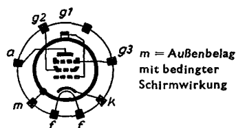
Sockelschaltschema
