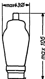
Kolbenabmessungen
