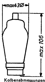
Kolbenabmessungen
