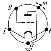
Sockelschalt-schema
