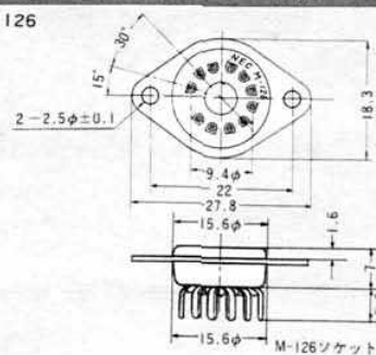
M-126 ソケット
