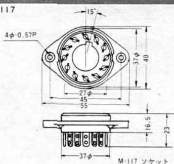
M-117 ソケット
