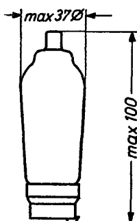
Kolbenabmessungen
