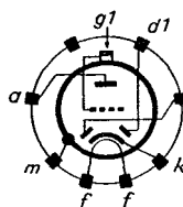
Sockelschaltschema
