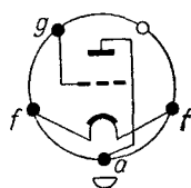
Sockelschaltschema
