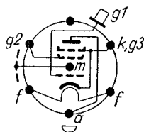
Sockelschaltchema
