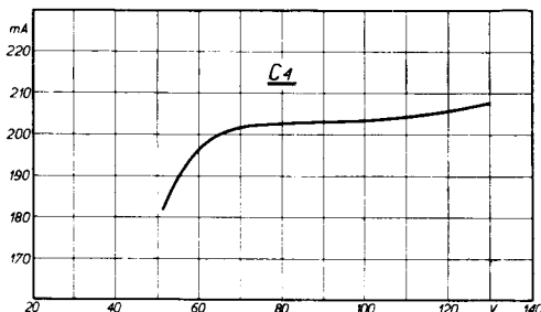
Kennlinie der Regulatorröhre C4. Der Regelbereich liegt zwischen 55 und 110 Volt.
