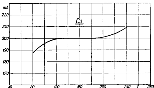
Kennlinie der Regulatorröhre C3. Der Regelbereich liegt zwischen 100 und 200 Volt.
