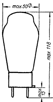
max. Abmessungen
