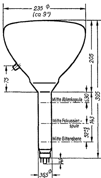
max. Abmessungen
