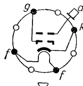
Sockelschaltchema
