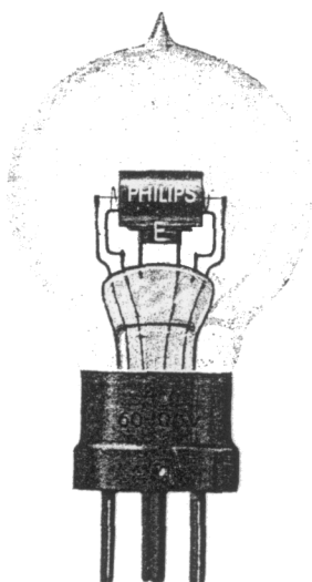
Abb. 5 Empfängerröhre Type E \frac{2}{3} der wirkl. Grösse
