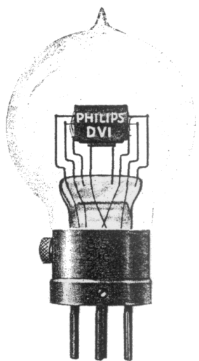
Abb. 7 Empfängerröhre Type D VI 2/3 der wirkl. Grösse
