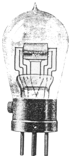
Abb. 6 Empfängerröhre Type B VI 2/3 der wirkl. Grösse
