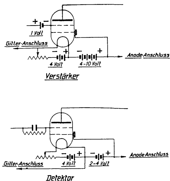
Abb. 8 Schaltungsbeispiele für type D VI.
