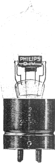
Abb. 2 Empfängerröhre Type D IV \frac{2}{3} der wirl. Grösse
