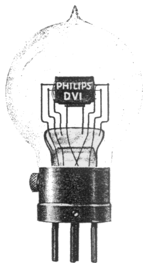
Abb. 7 Empfängerröhre Type D VI 2/3 der wirkl. Grösse
